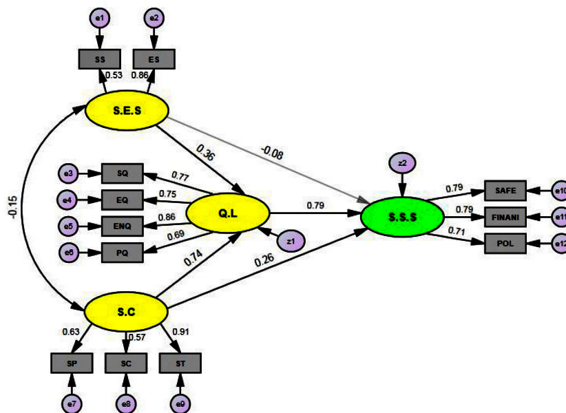
شکل ۳: ضرایب رگرسیونی استاندارد مدل پیشنهادی پژوهش (منبع: یافته‌های پژوهش، ۱۳۹۶)
