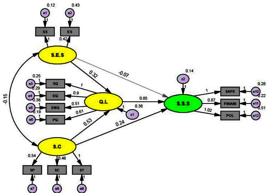
شکل ۲: ضرایب رگرسیونی غیراستاندارد مدل پیشنهادی پژوهش (منبع: یافته‌های پژوهش، ۱۳۹۶)
