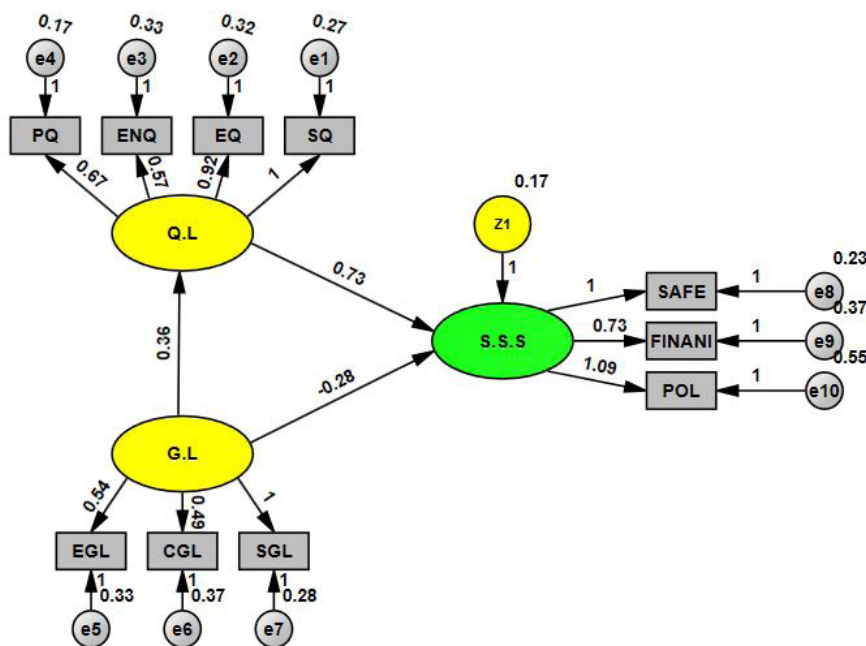
شکل ۲: ضرایب رگرسیونی غیراستاندارد الگوی پیشنهادی پژوهش (منبع: یافته‌های تحقیق، ۱۳۹۸)
