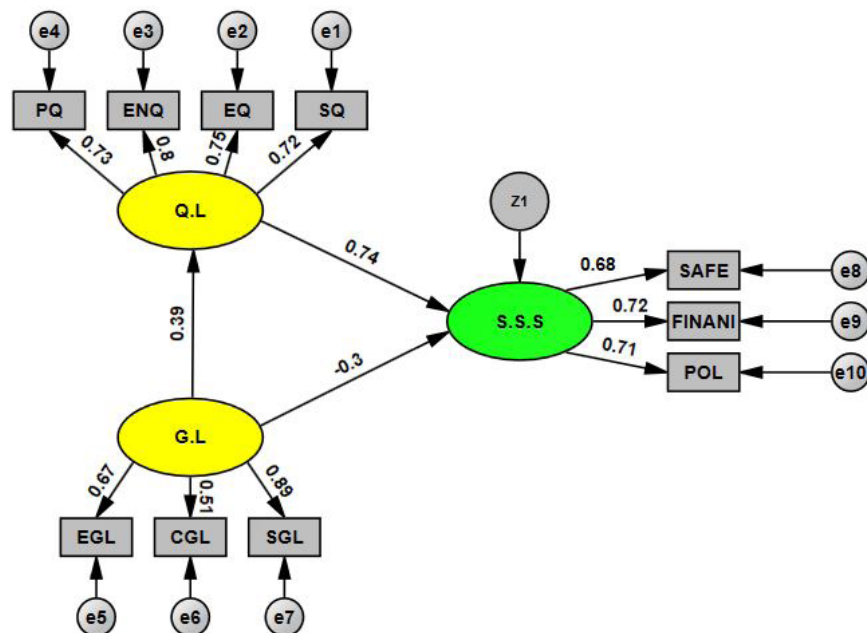
شکل ۳: ضرایب رگرسیونی استاندارد الگوی پیشنهادی پژوهش (منبع: یافته‌های تحقیق، ۱۳۹۸)
